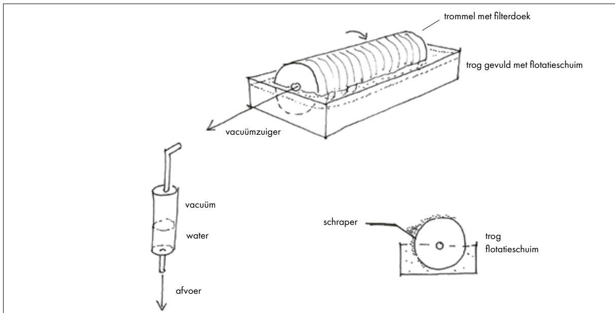
vacuüm trommelfilter
